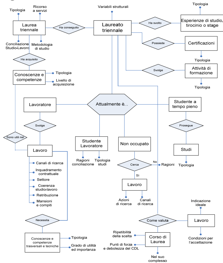
Figura. 2 Schema Entità-Relazione
